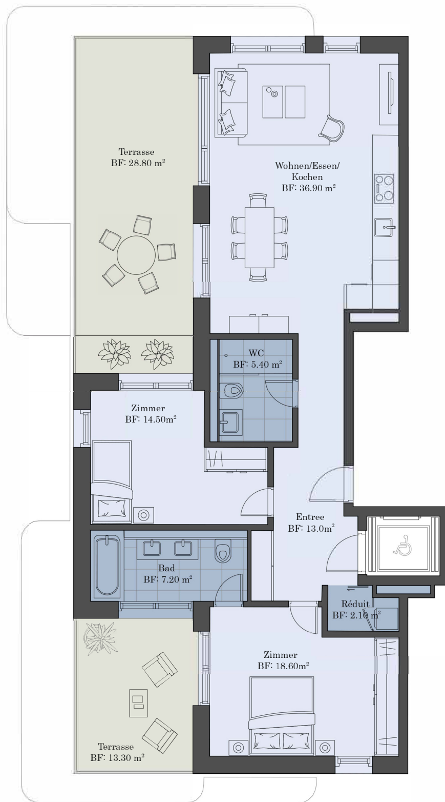
HAUS B - WHG 8 Attikageschoss Wohnfläche 101.80 m 2
